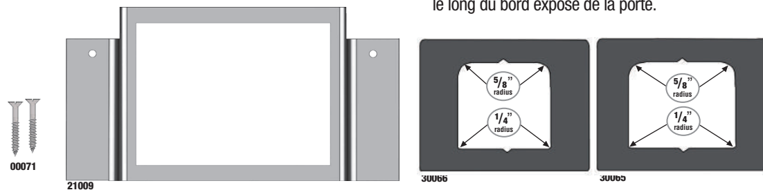
Easy Measuring Guide for 3" and 3 1/2" Hinges • Guía de medición fácil para bisagras de 3" y 3 1/2" pulgadas • Guide de mesurage facile pour les charnières de 3" et 3,5" po
